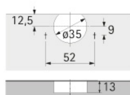
Cotes de perçage TX32/52x9 Selekt Pro 2000
