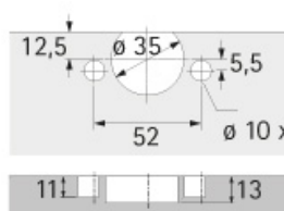
Cotes de perçage TH33 Selekt Pro 2000
