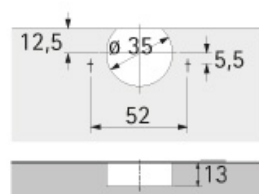
Cotes de perçage TH32 Selekt Pro 2000
