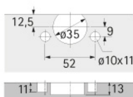
Cotes de perçage TX33/52x9 Selekt Pro 2000
